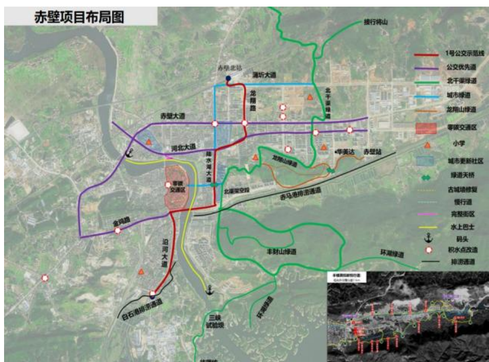
图 1-1 赤壁市项目布局图
